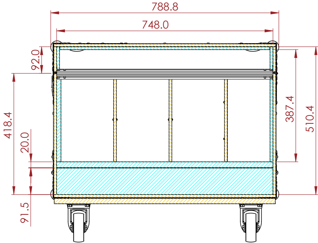
SECTION B-B SCALE 1 : 8
